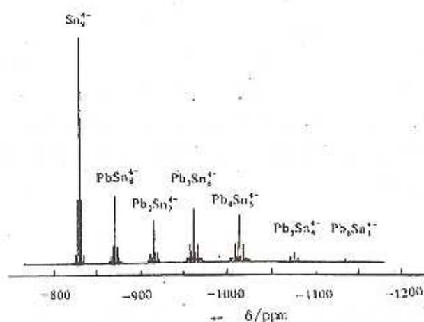
图 1 K_4Pb_xSn_{(9-x)} 体系的 ^{119}Sn NMR 谱
