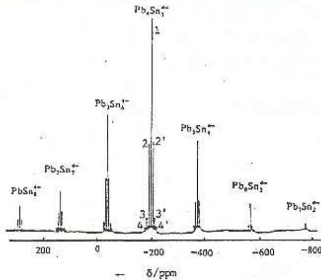
图2 K_4Pb_xSn_{(9-x)} 体系的 ^{207}Pb NMR 谱 Fig.2 ^{207}Pb NMR spectrum of the system K_4Pb_xSn_{(9-x)}
